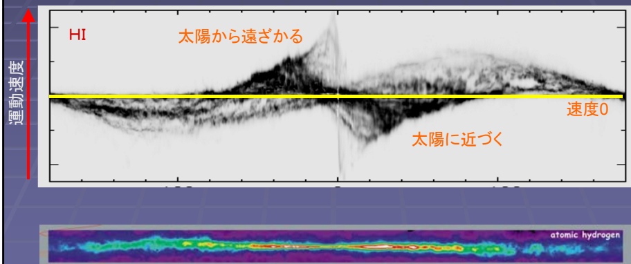
水素ガスの分布図
