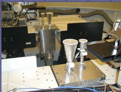
VERAの受信機 (22GHz & 43 GHz)
