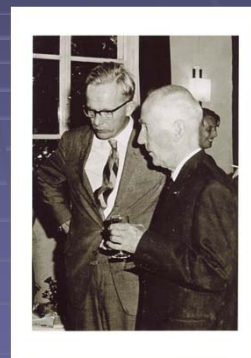
中性水素21cmを予言した Jan Oort (1900 - 1992) Hendrik van de Hulst (1918-2000)
